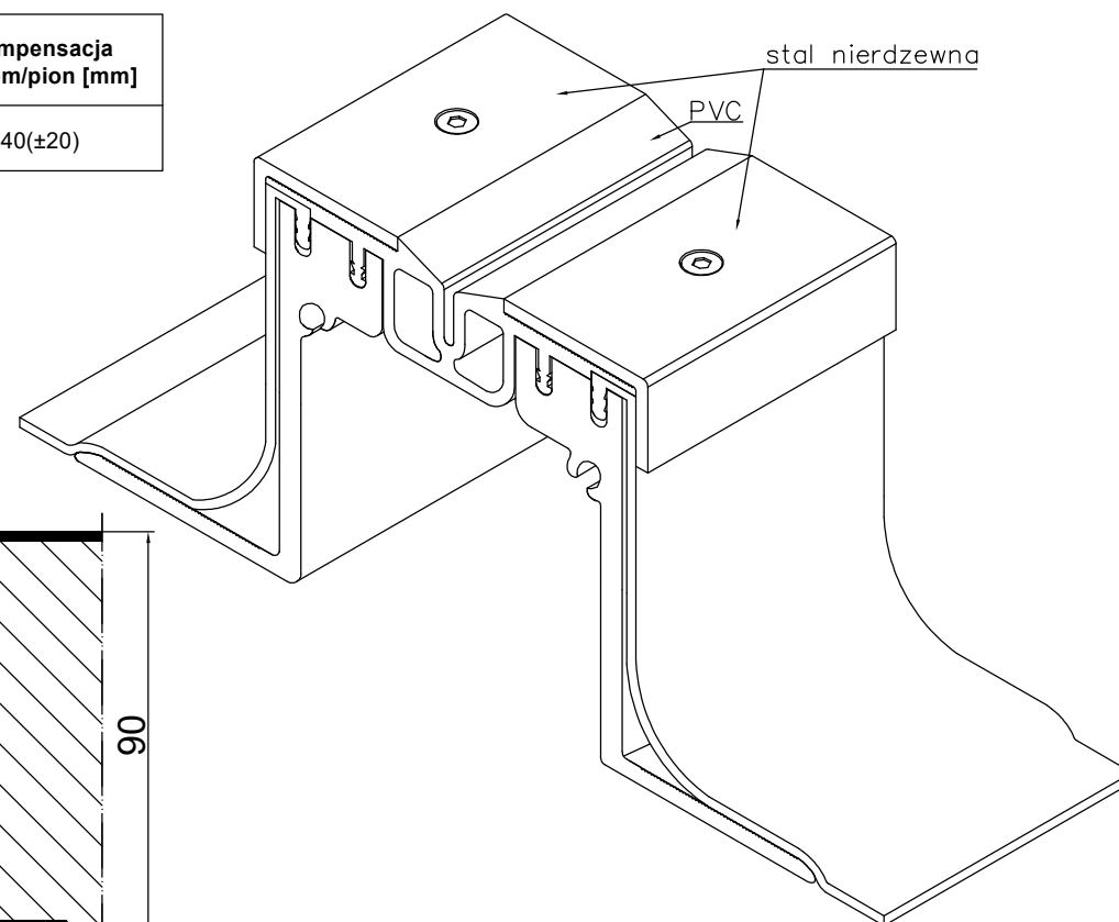
CONECTO GA 50.20.90 L Rzut aksonometryczny
