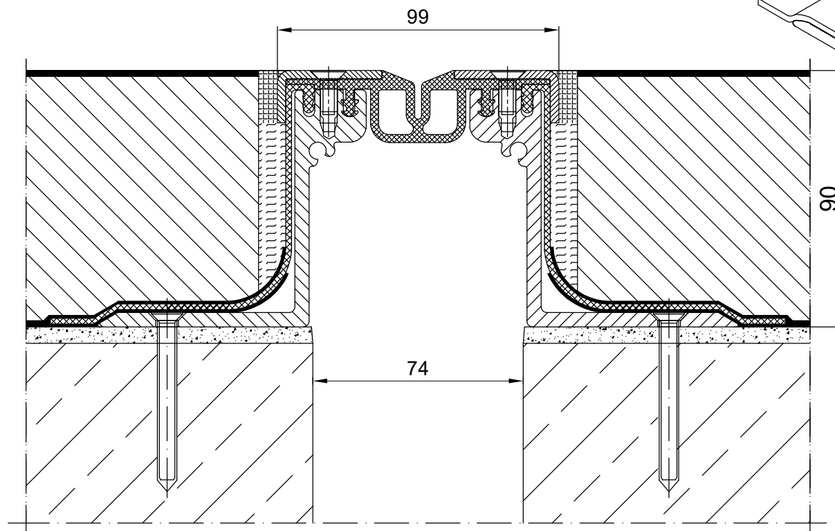
CONECTO GA 50.20.90 L Przekrój
