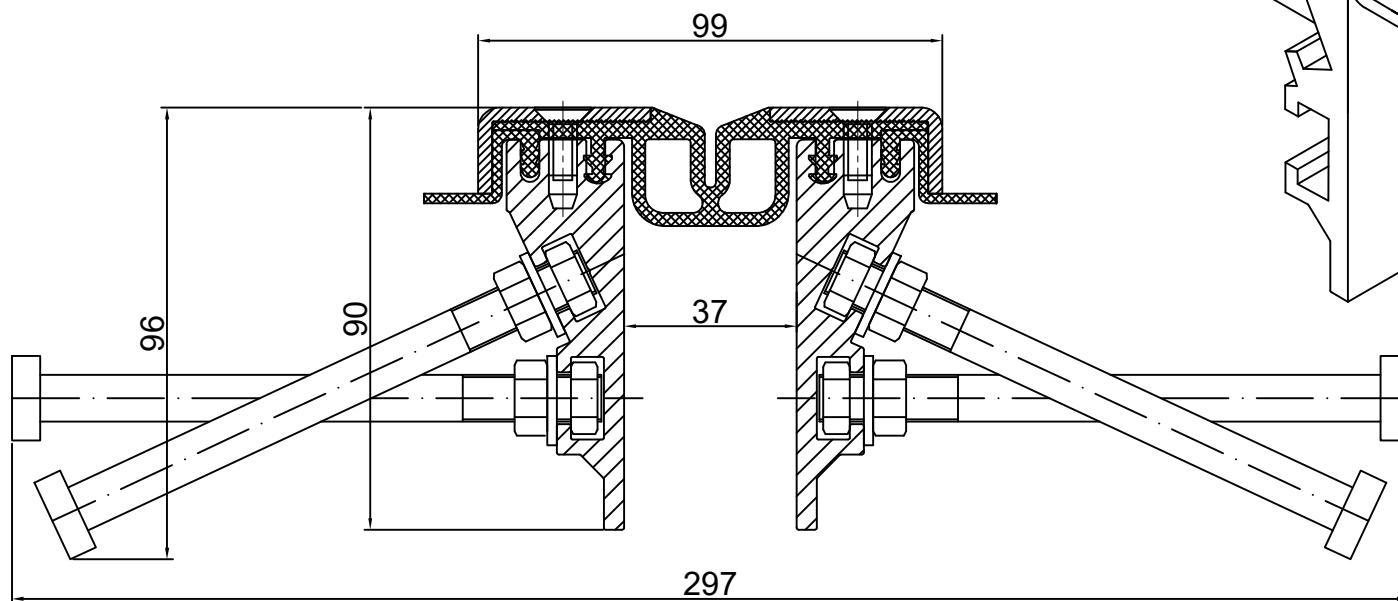
CONECTO GA 50.20.90& S PRZEKRÓJ
