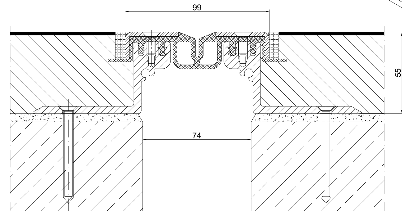
PROFIL DYLATACJNY GA 50.20.55 S PRZEKRÓJ
