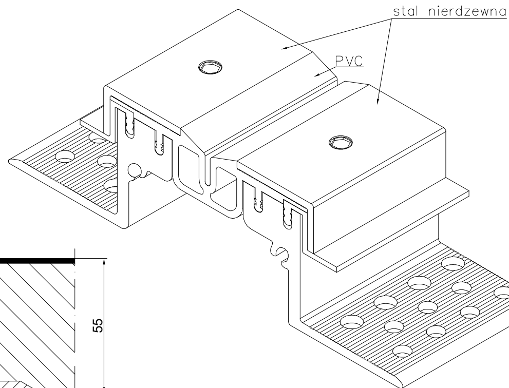
PROFIL DYLATACJNY GA 50.20.55 S RZUT AKSONOMETRYCZNY
