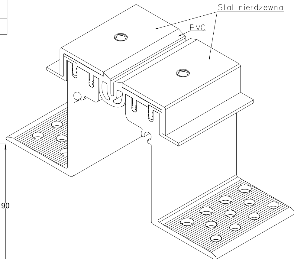
CONECTO GA 43.10.90 S RZUT AKSONOMETRYCZNY
