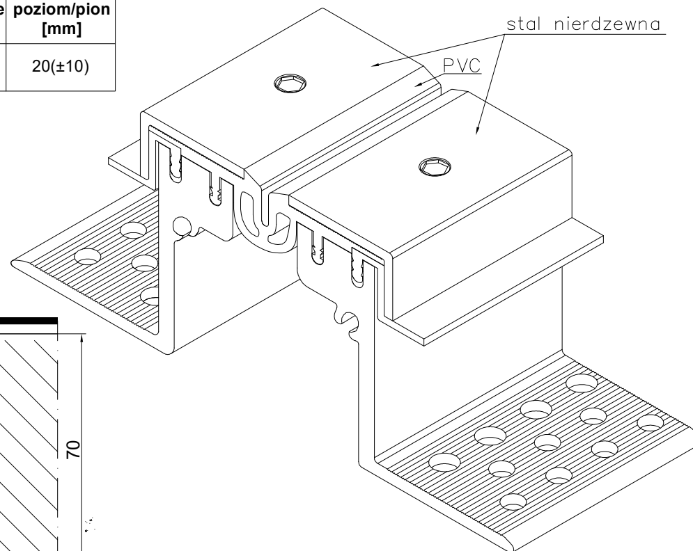
CONECTO GA 43.10.70 S RZUT AKSONOMETRYCZNY
