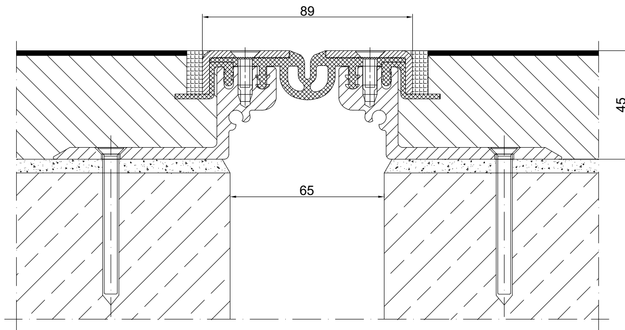
PROFIL DYLATACJNY GA 43.10.45 S PRZEKRÓJ
