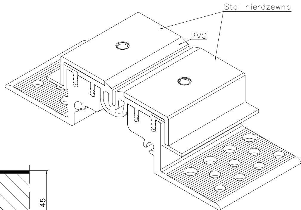
PROFIL DYLATACJNY GA 43.10.45 S RZUT AKSONOMETRYCZNY
