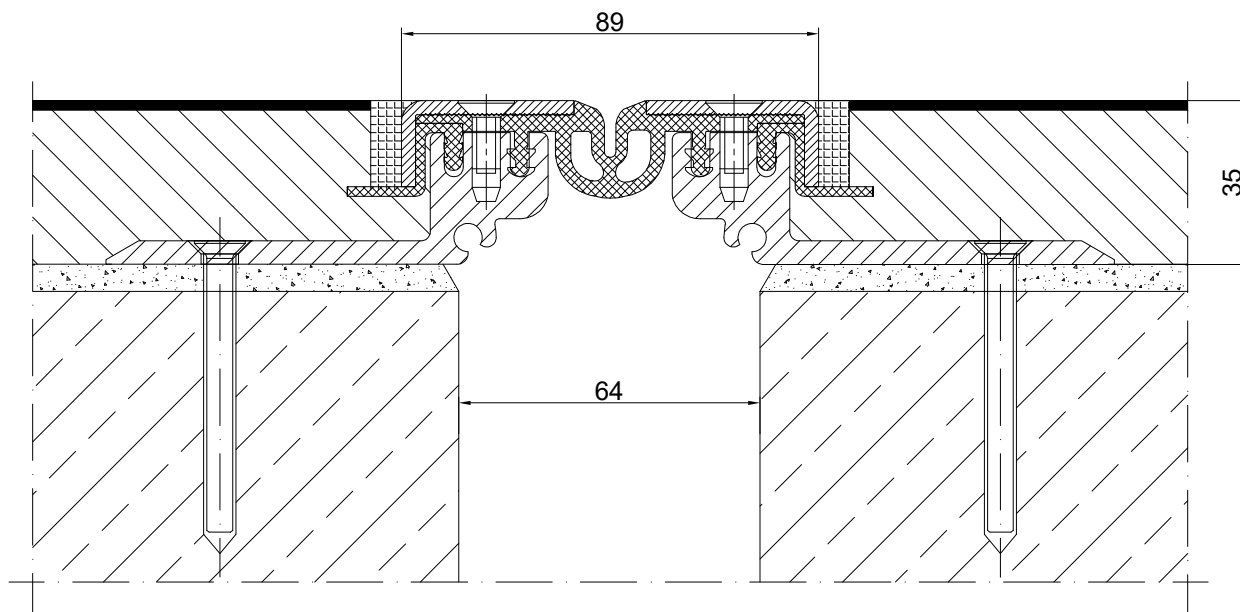
PROFIL DYLATACJNY GA 43.10.35 S PRZEKRÓJ
