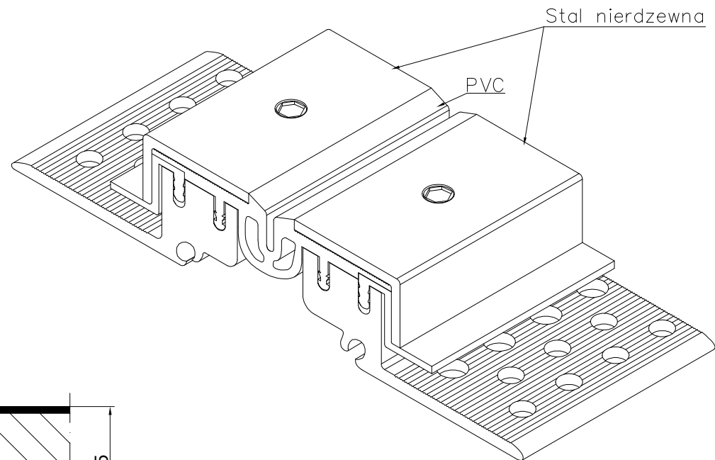
PROFIL DYLATACJNY GA 43.10.35 S RZUT AKSONOMETRYCZNY
