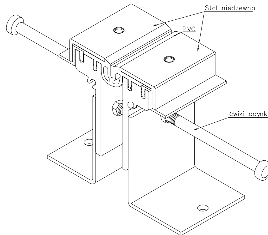
CONECTO PARK GA 43.10.120& S z ocynkowanymi ćwikami RZUT AKSONOMETRYCZNY
