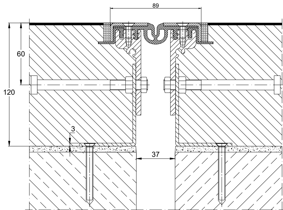
CONECTO PARK GA 43.10.120& S z ocynkowanymi ćwikami PRZEKRÓJ
