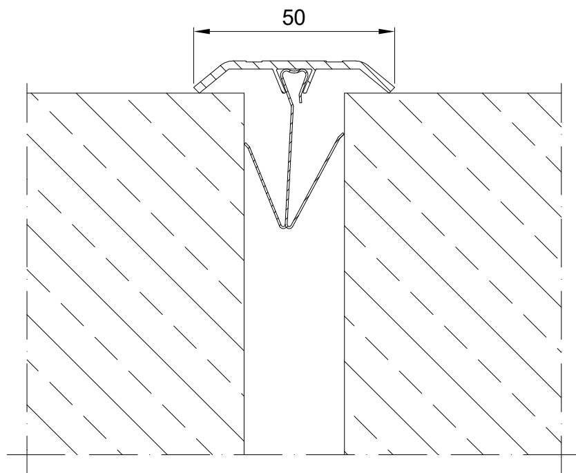
PROFIL DYLATACJNY JW 50 PRZEKRÓJ
