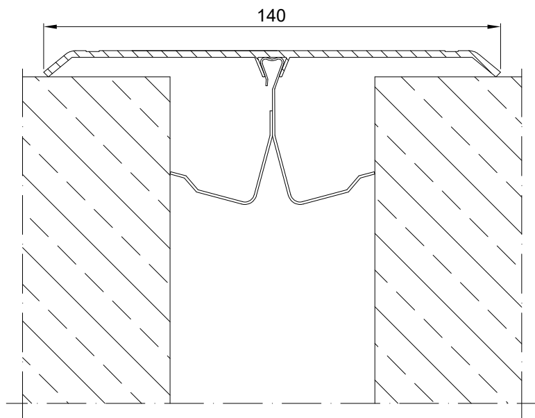
PROFIL DYLATACJNY JW 140 PRZEKRÓJ
