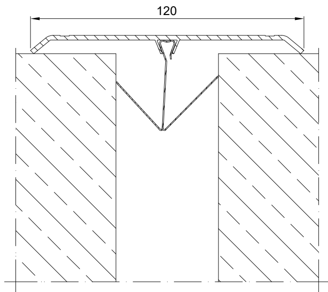
PROFIL DYLATACJNY JW 120 PRZEKRÓJ
