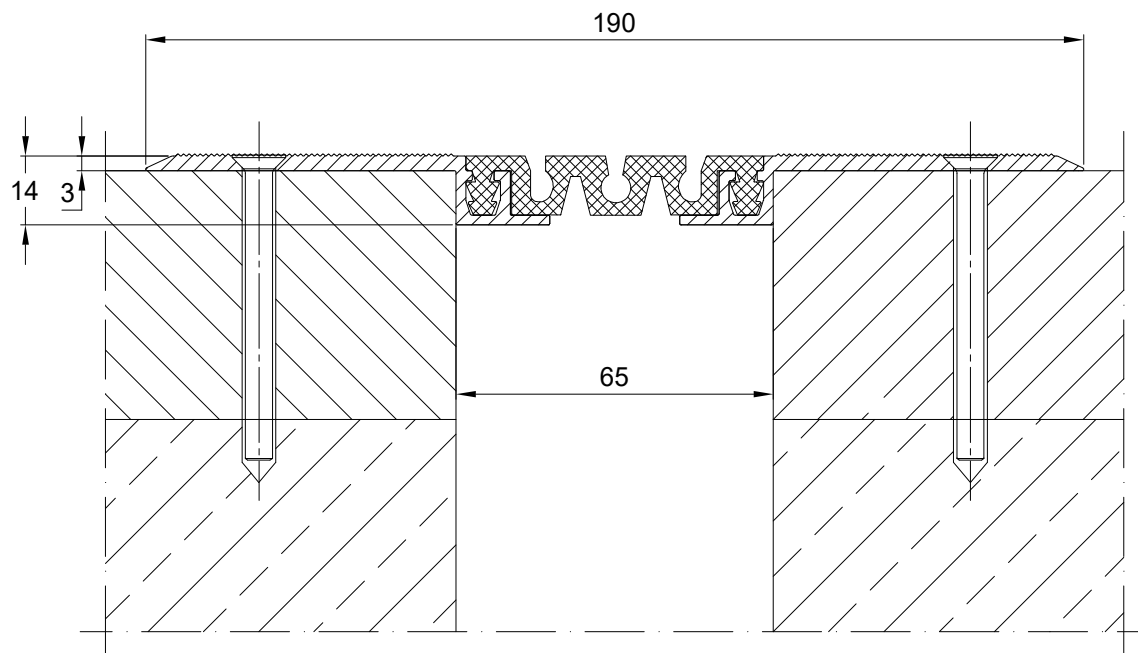
PROFIL DYLATACJNY EL 65.10 N PRZEKRÓJ
