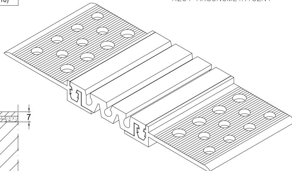
PROFIL DYLATACJNY EL 65.10.7 RZUT AKSONOMETRYCZNY
