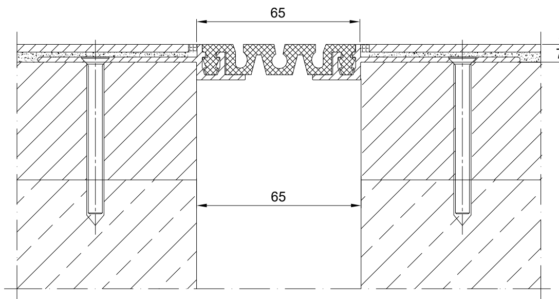
PROFIL DYLATACJNY EL 65.10.7 PRZEKRÓJ
