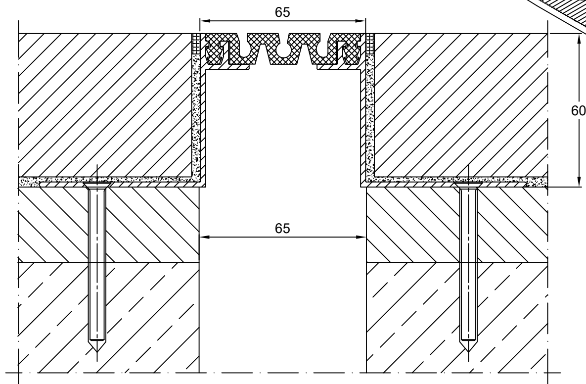
PROFIL DYLATACJNY EL 65.10.60 PRZEKRÓJ
