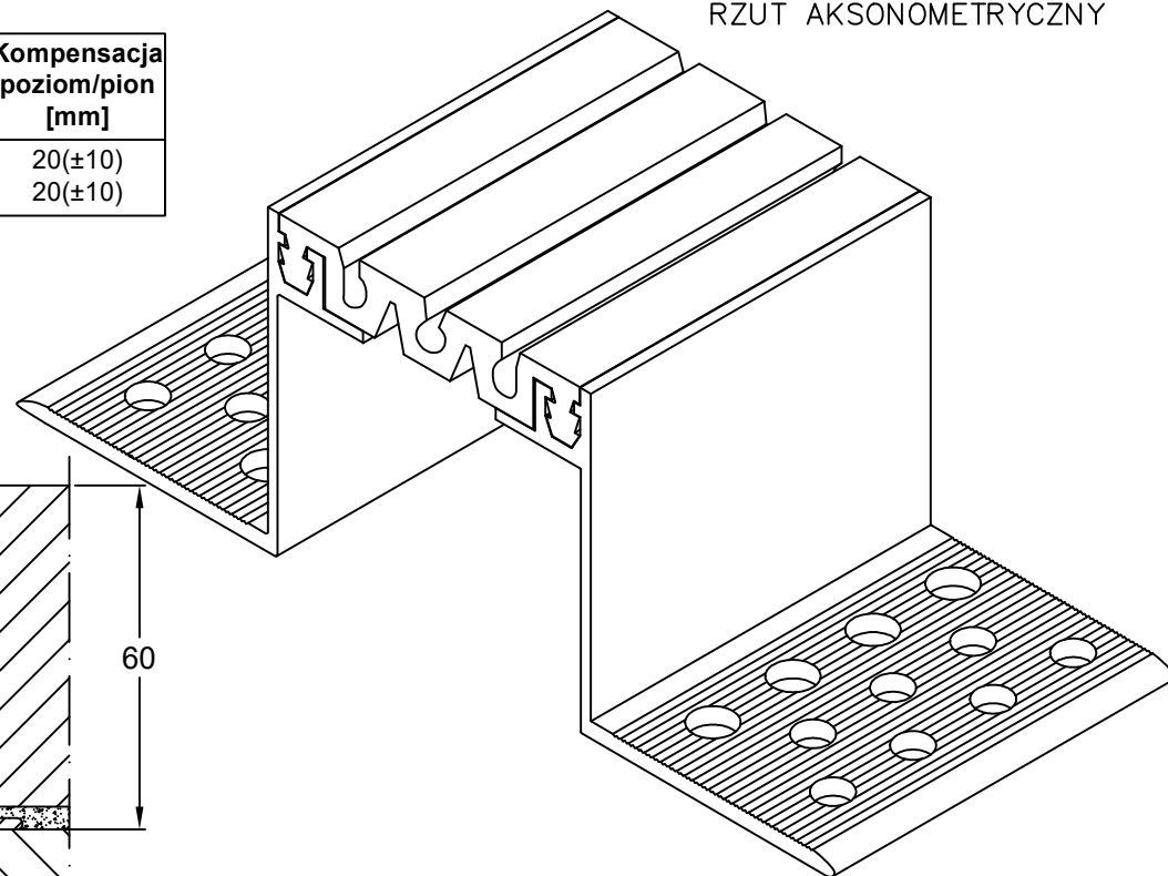
PROFIL DYLATACJNY EL 65.10.60 RZUT AKSONOMETRYCZNY
