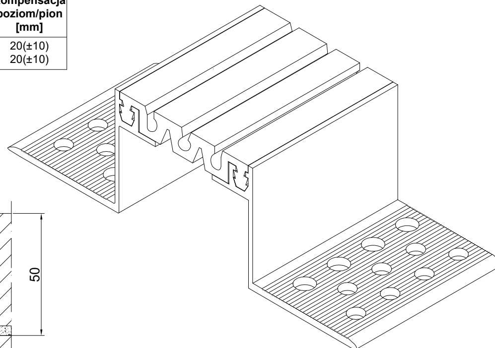
PROFIL DYLATACJNY EL 65.10.50 RZUT AKSONOMETRYCZNY
