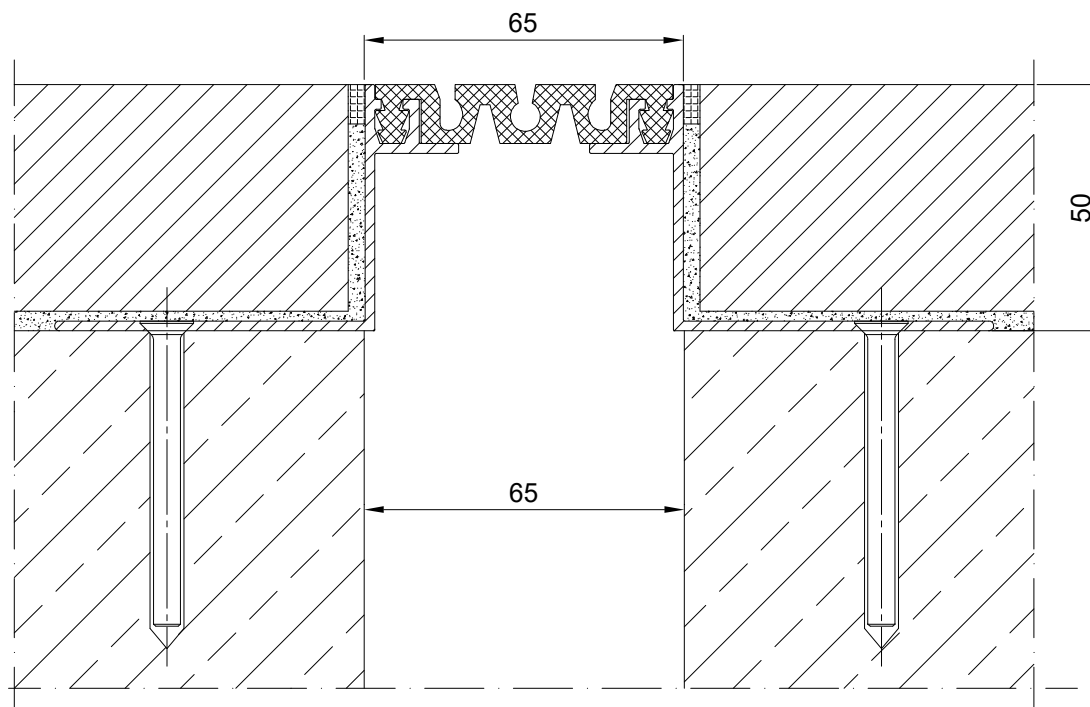
PROFIL DYLATACJNY EL 65.10.50 PRZEKRÓJ
