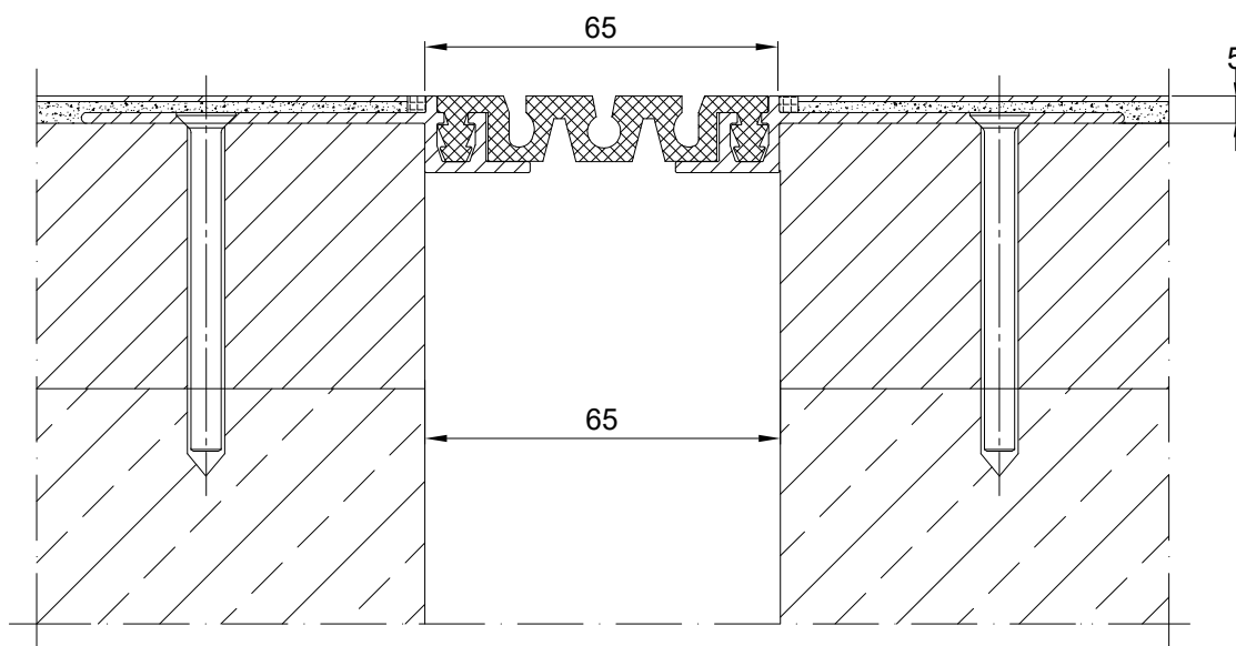
PROFIL DYLATACJNY EL 65.10.5 PRZEKRÓJ
