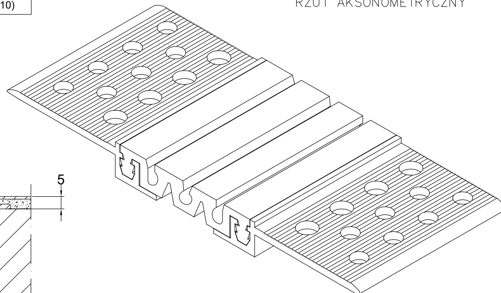
PROFIL DYLATACJNY EL 65.10.5 RZUT AKSONOMETRYCZNY
