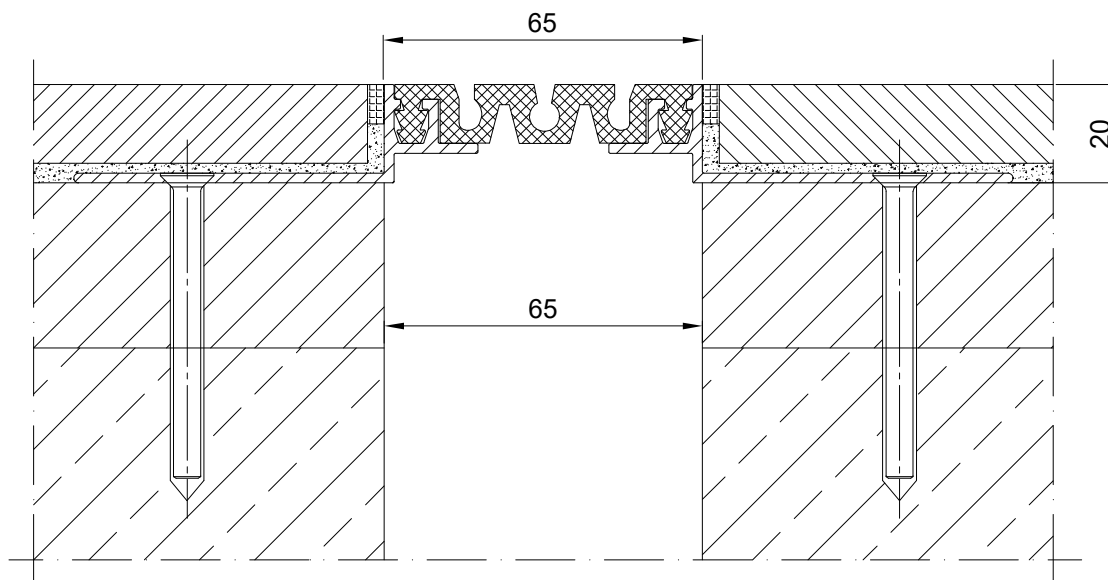
PROFIL DYLATACJNY EL 65.10.20 PRZEKRÓJ
