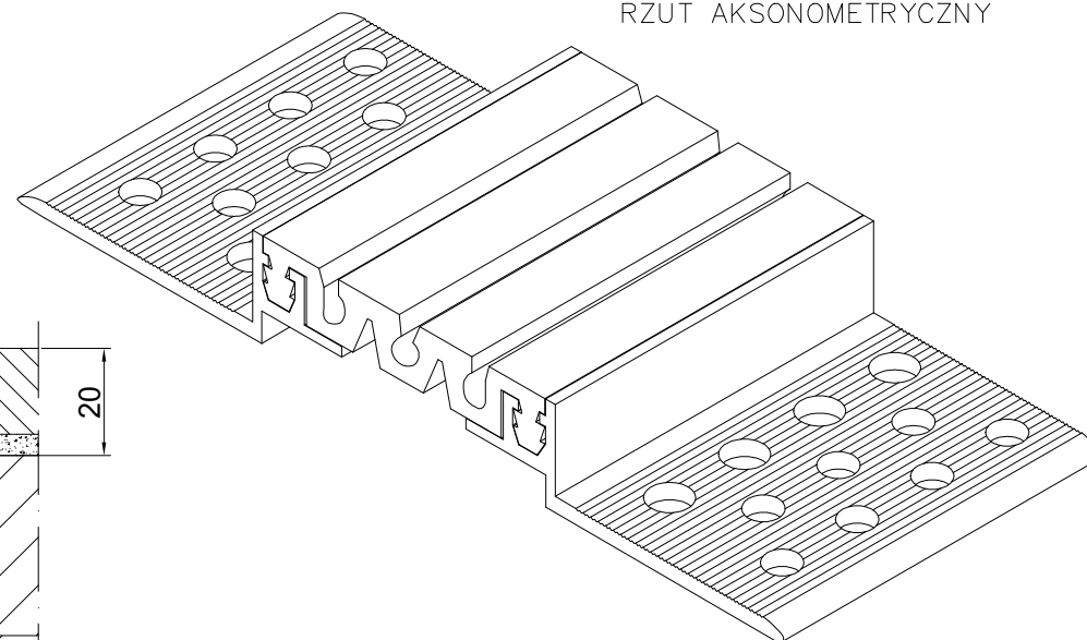
PROFIL DYLATACJNY EL 65.10.20 RZUT AKSONOMETRYCZNY
