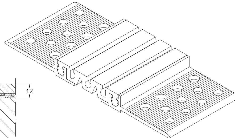
PROFIL DYLATACJNY EL 65.10.12 RZUT AKSONOMETRYCZNY
