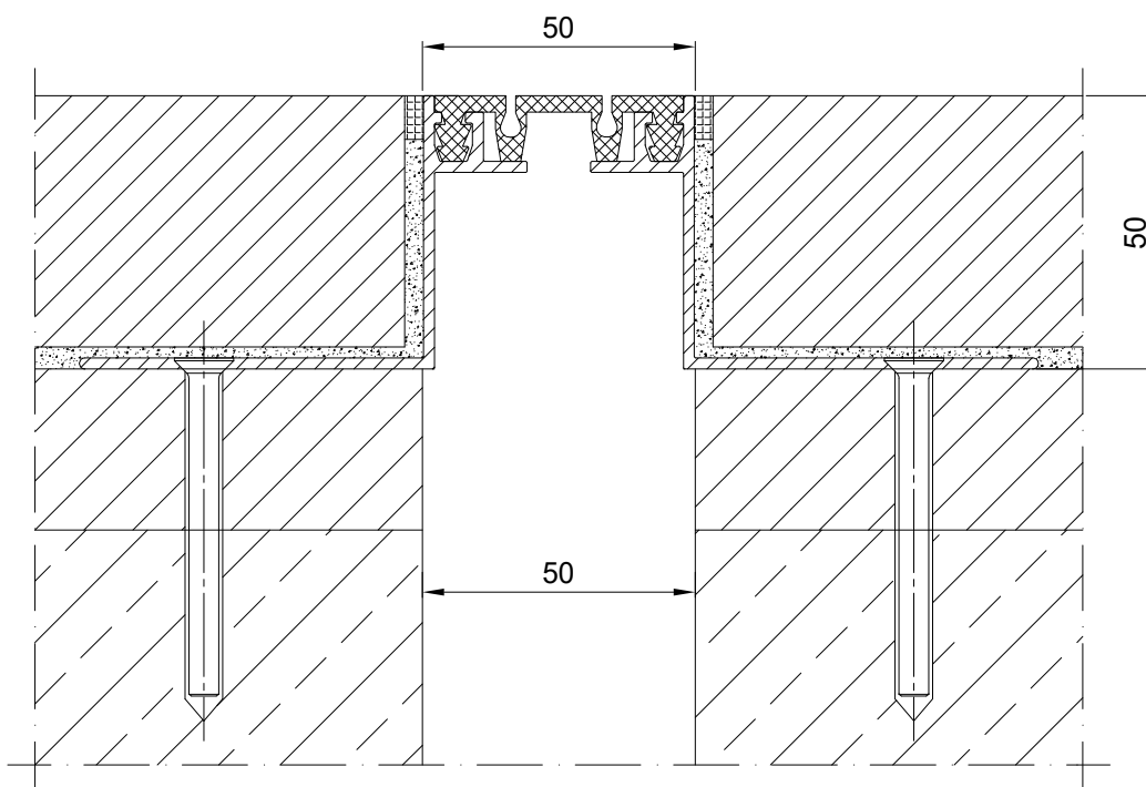
PROFIL DYLATACJNY EL 50.8.50 PRZEKRÓJ
