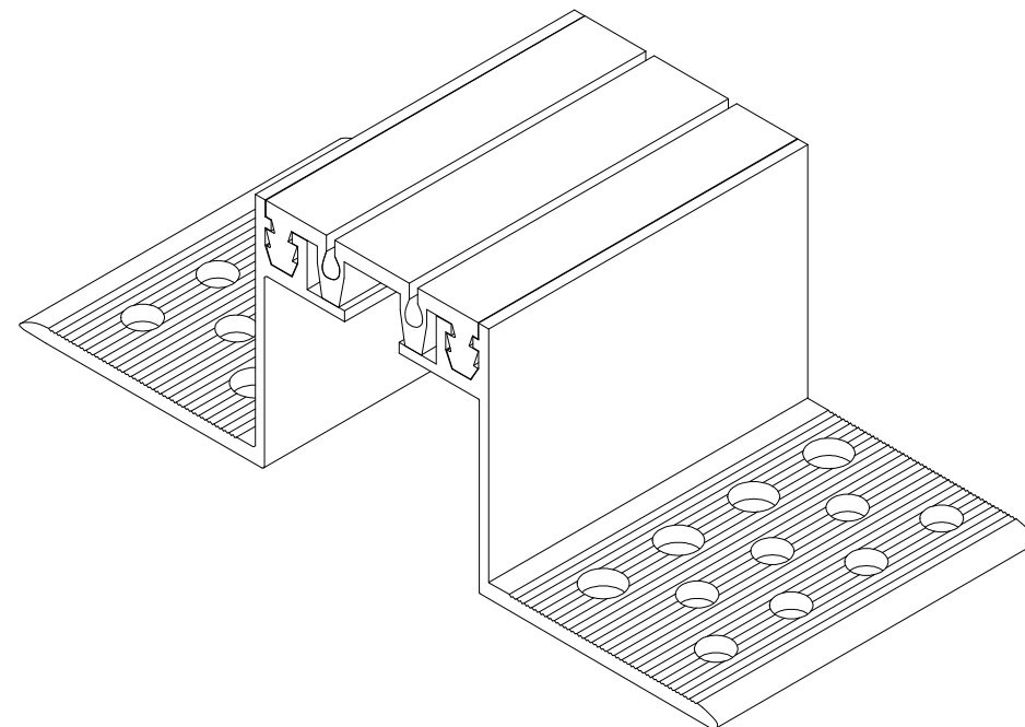
PROFIL DYLATACJNY EL 50.8.50 RZUT AKSONOMETRYCZNY
