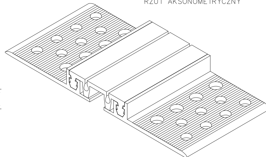
PROFIL DYLATACJNY EL 50.8.14 RZUT AKSONOMETRYCZNY
