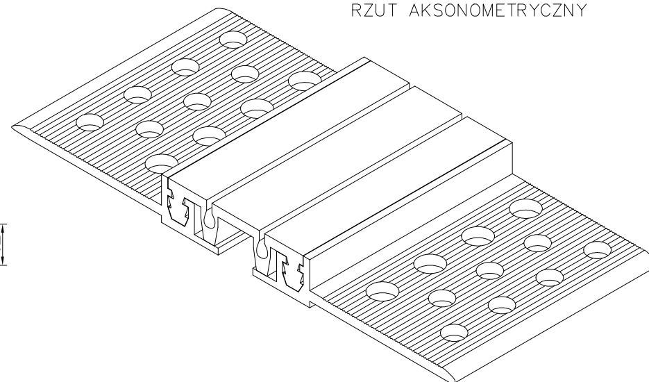
PROFIL DYLATACJNY EL 50.8.12 RZUT AKSONOMETRYCZNY
