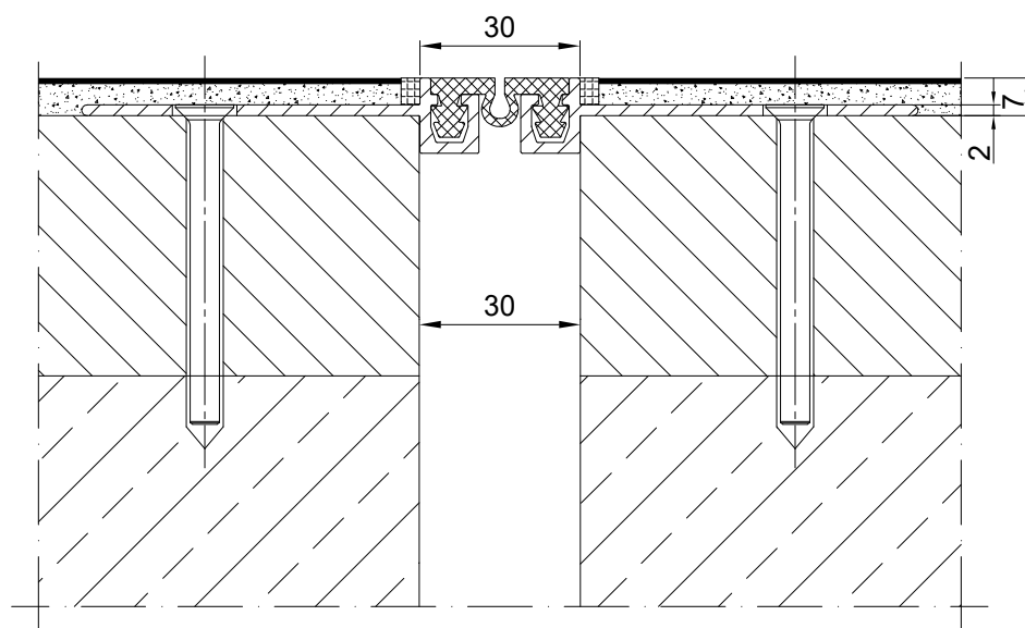
PROFIL DYLATACJNY EL 30.6.7 PRZEKRÓJ
