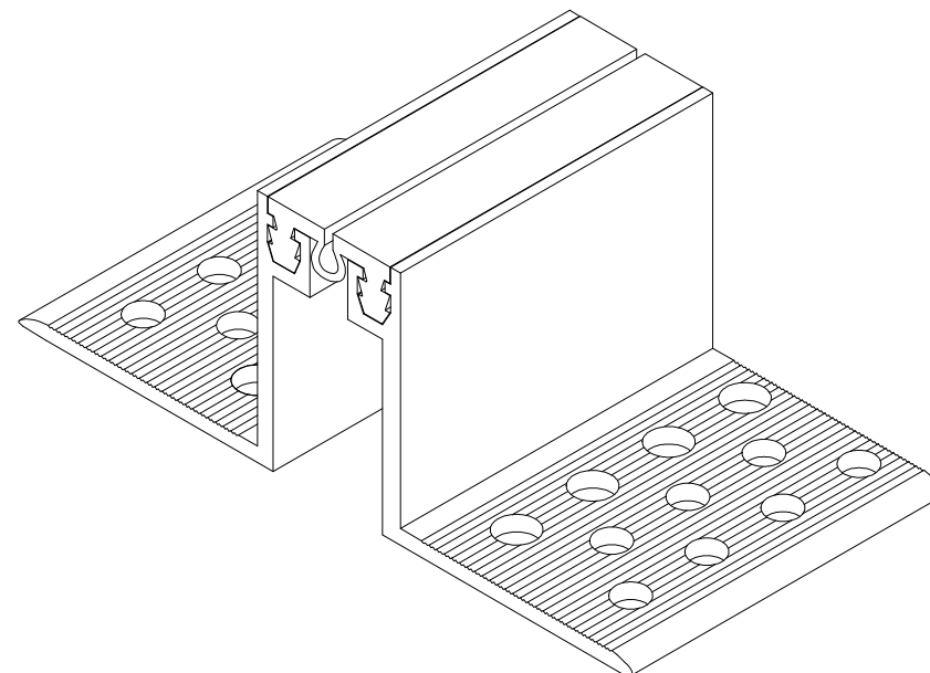
CONECTO EL 30.6.50 RZUT AKSONOMETRYCZNY
