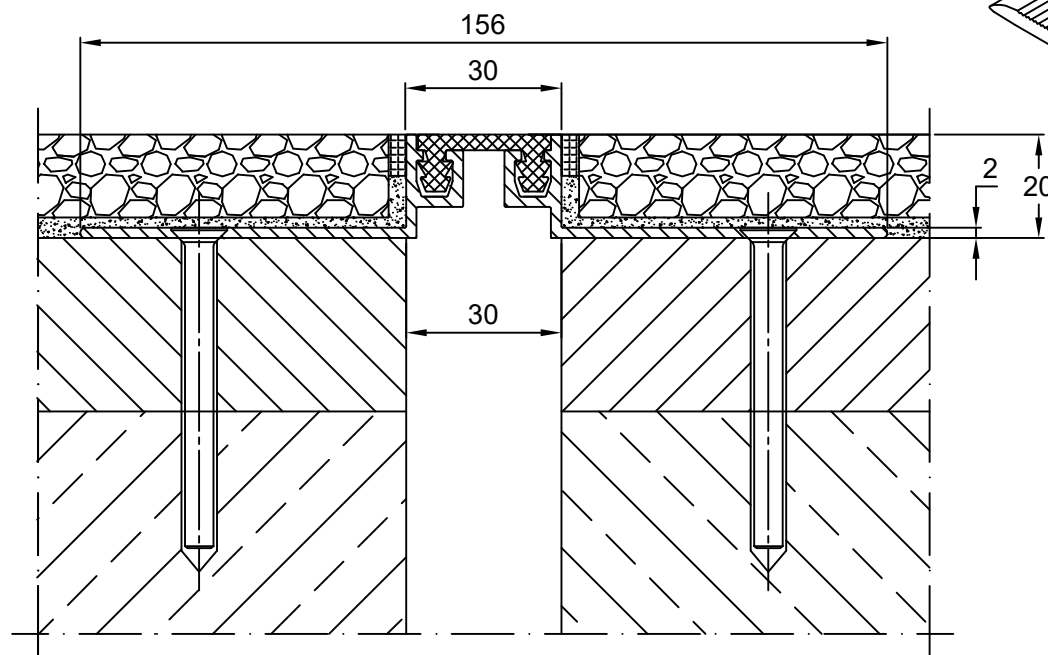
CONECTO EL 30.6.20 Przekrój
