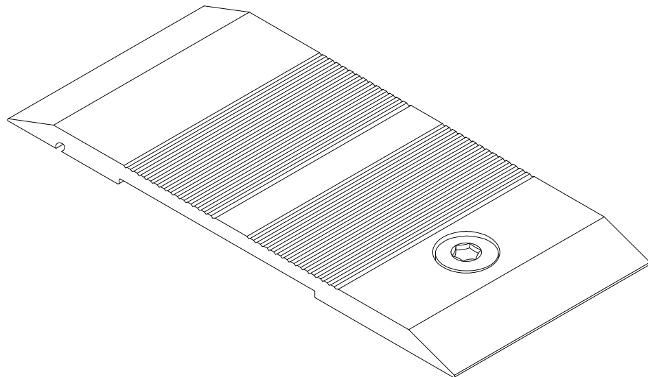
PROFIL DYLATACJNY CS 160 RZUT AKSONOMETRYCZNY
