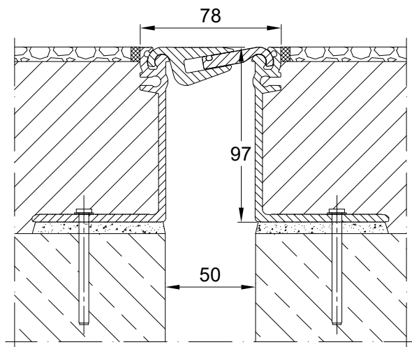
PROFIL DYLATACJNY AL 78.10.97 PRZEKRÓJ SKALA 1:2
