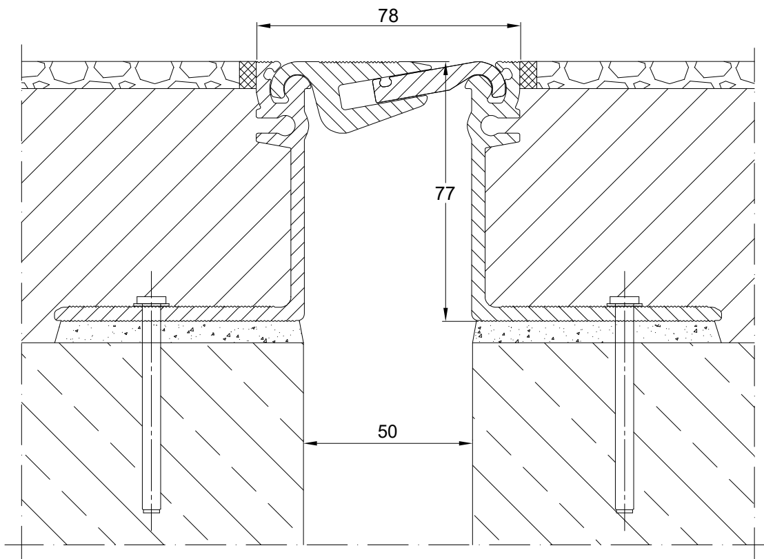
CONECTO AL 78.10.77 PRZEKRÓJ
