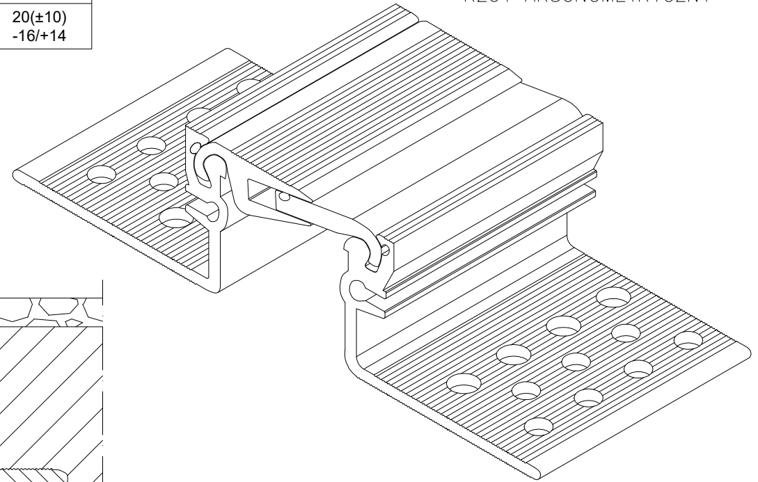
PROFIL DYLATACJNY AL 78.10.52 RZUT AKSONOMETRYCZNY
