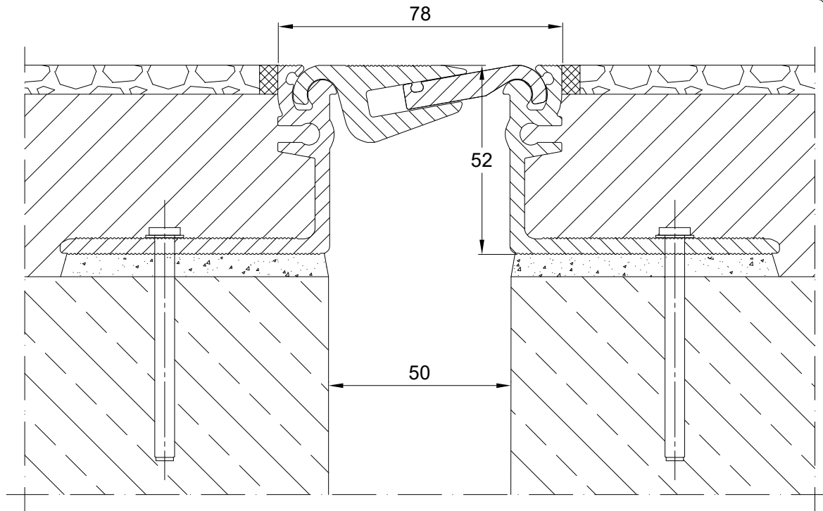
PROFIL DYLATACJNY AL 78.10.52 PRZEKRÓJ
