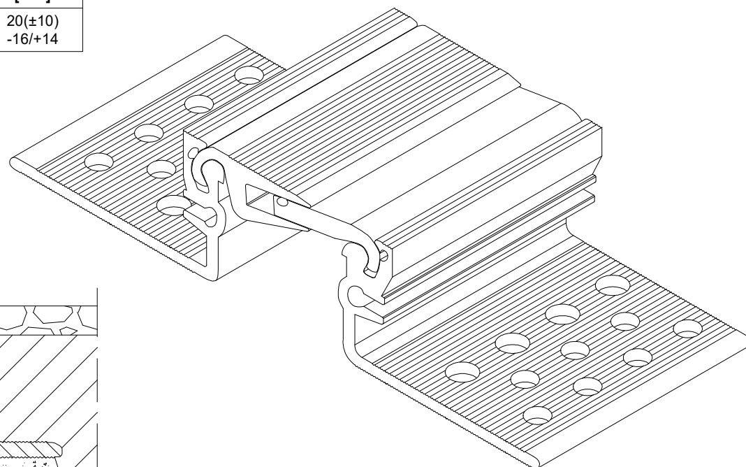
PROFIL DYLATACYJNY AL 78.10.42 RZUT AKSONOMETRYCZNY
