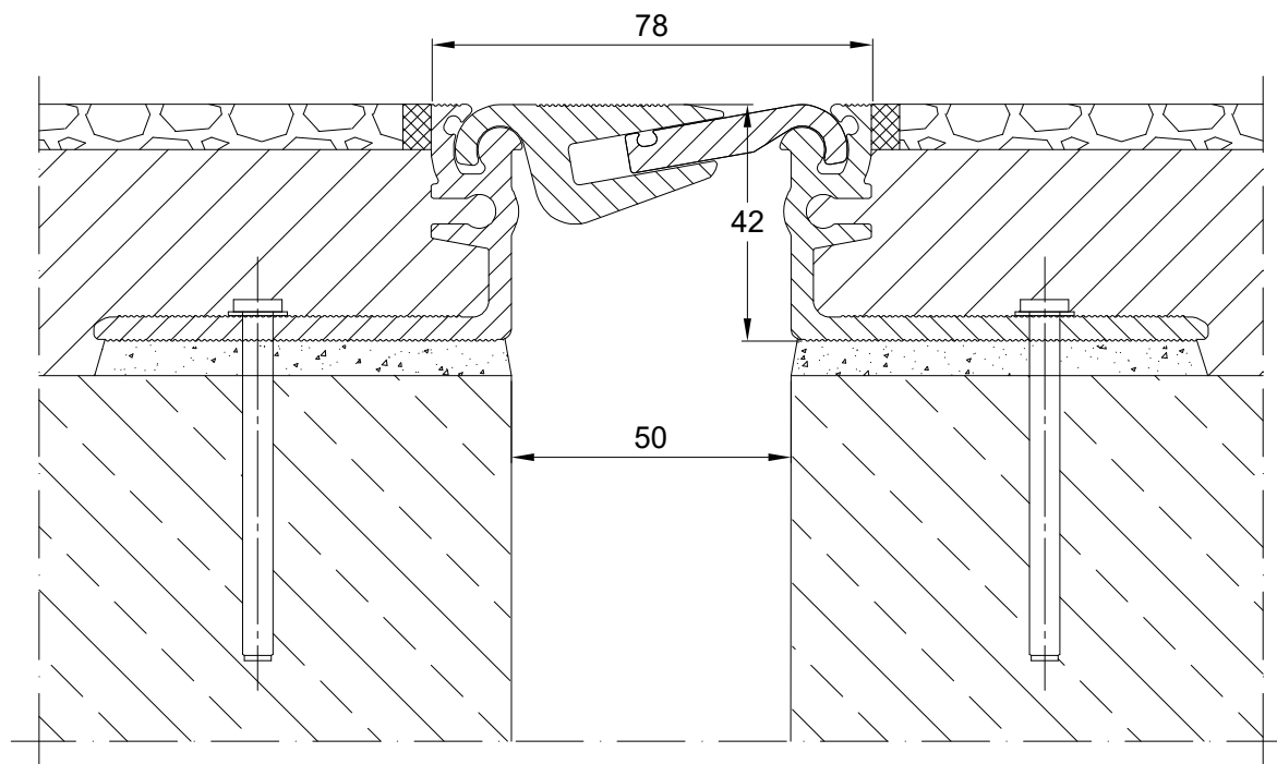
PROFIL DYLATACYJNY AL 78.10.42 PRZEKRÓJ
