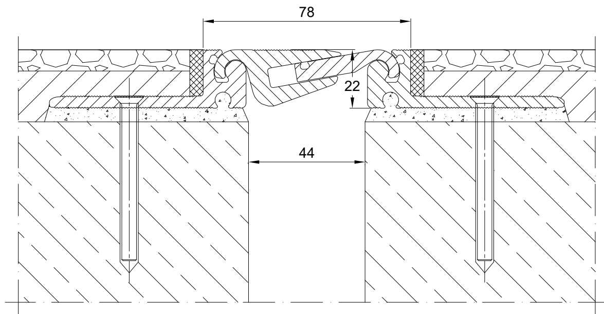
PROFIL DYLATACJNY AL 78.10.22 PRZEKRÓJ
