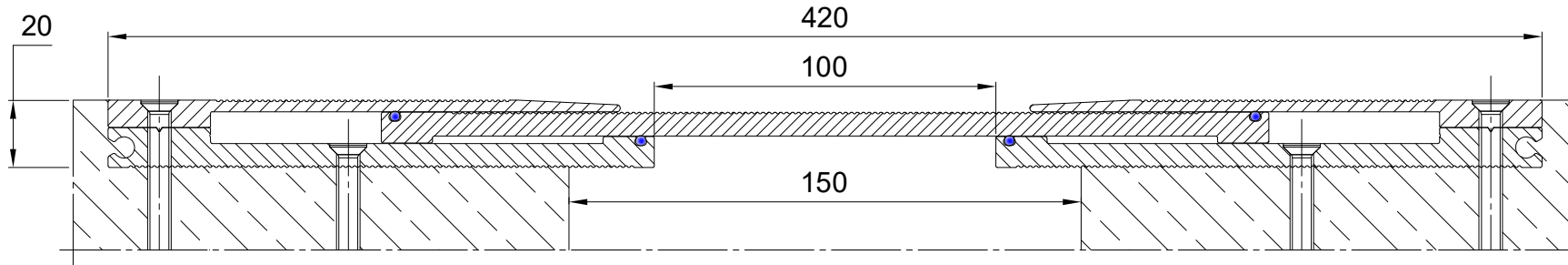
Conecto AL 420 PRZEKRÓJ SKALA 1:1,75
