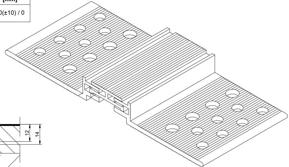
PROFIL DYLATACJNY AL 38.10.14 RZUT AKSONOMETRYCZNY
