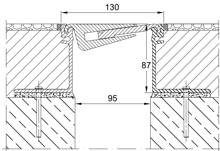
PROFIL DYLATACJNY AL 130.21.87 PRZEKRÓJ SKALA 1:2
