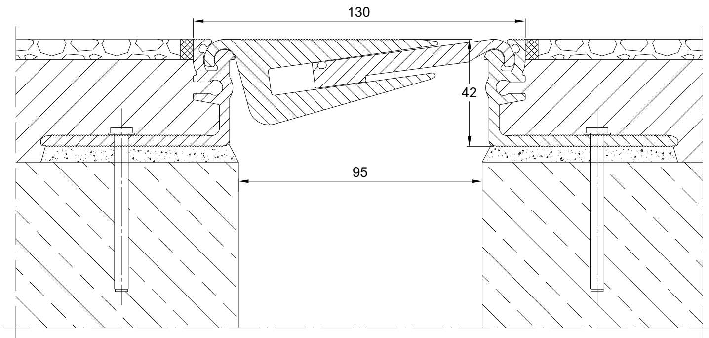
PROFIL DYLATACJNY AL 130.21.42 PRZEKRÓJ
