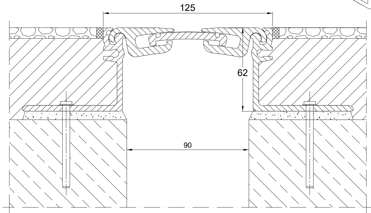
CONECTO AL 125.20.62 PRZEKRÓJ
