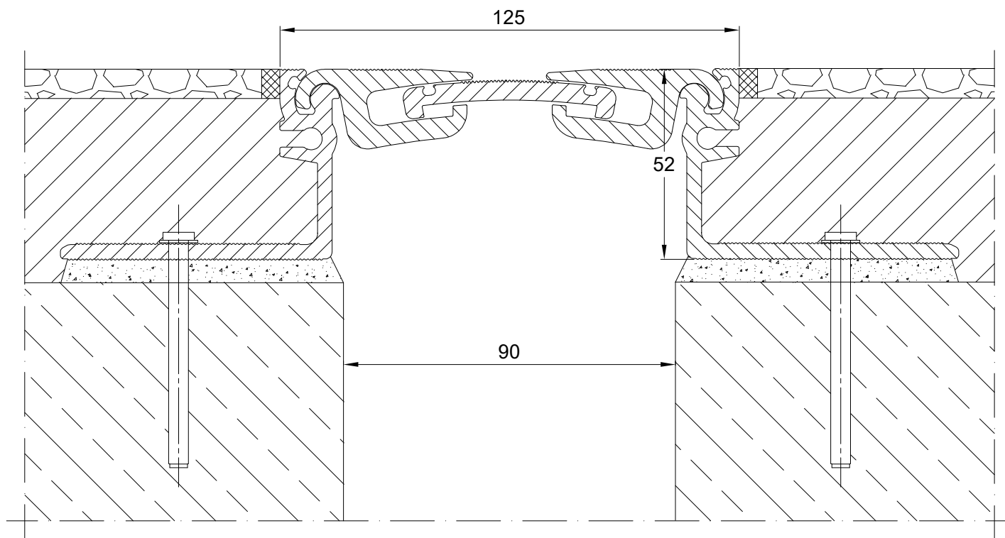
PROFIL DYLATACJNY AL 125.20.52 PRZEKRÓJ
