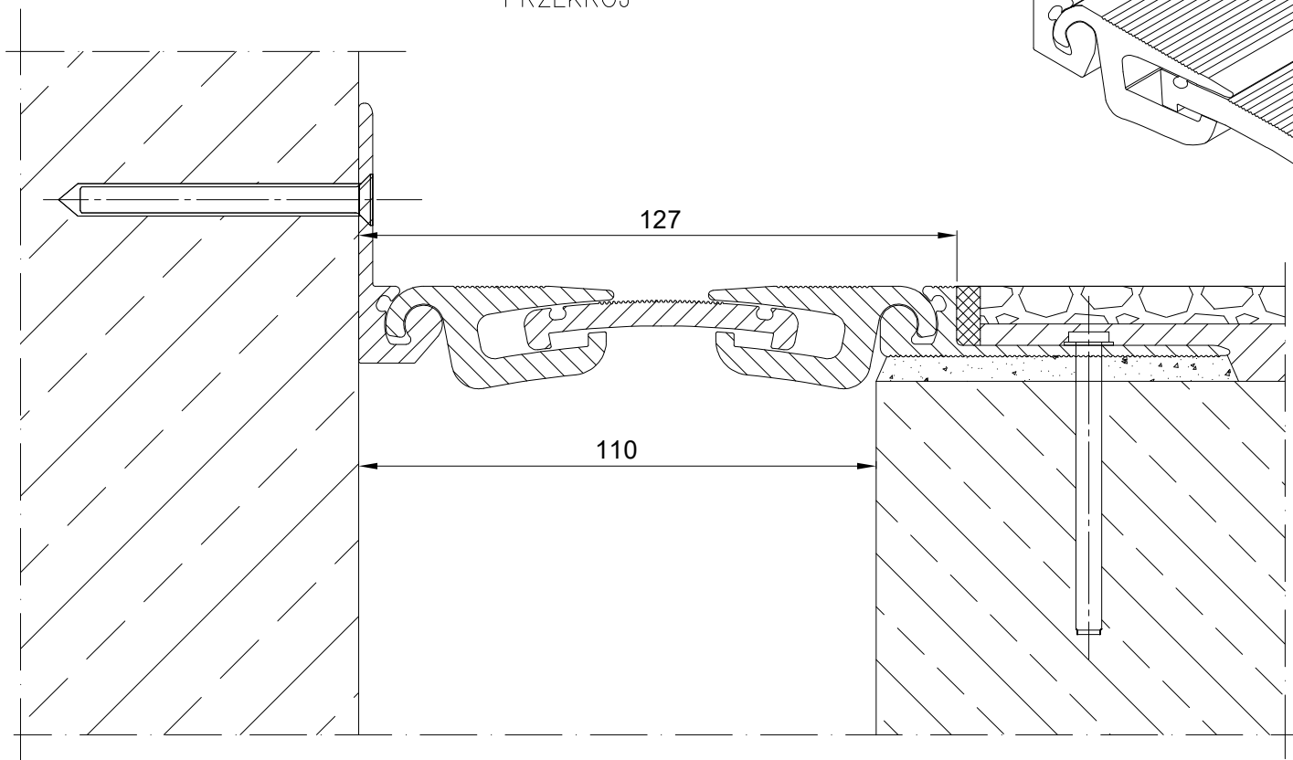
PROFIL DYLATACJNY AL 125.20.15 CV PRZEKRÓJ
