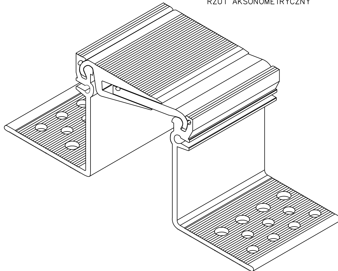
PROFIL DYLATACJNY AL 110.15.97 RZUT AKSONOMETRYCZNY
