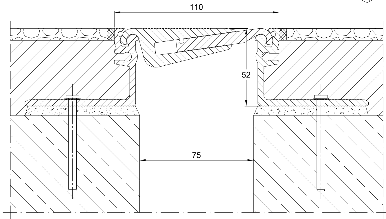
PROFIL DYLATACJNY AL 110.15.52 PRZEKRÓJ
