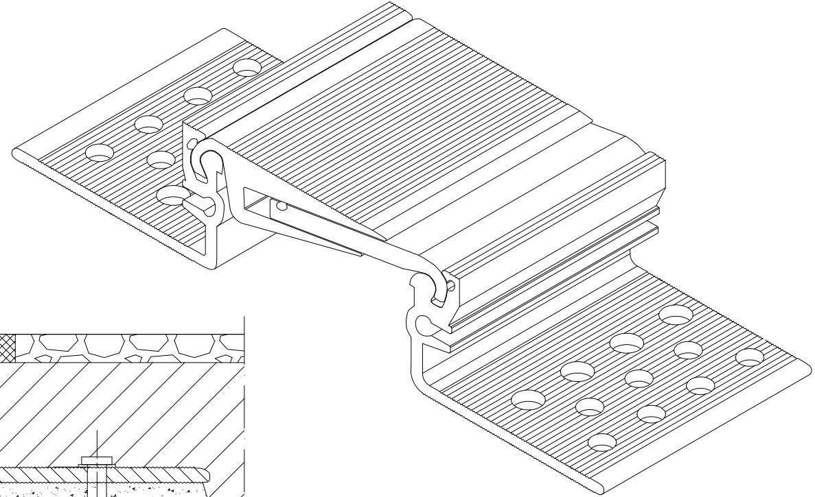
PROFIL DYLATACJNY AL 110.15.42 RZUT AKSONOMETRYCZNY
