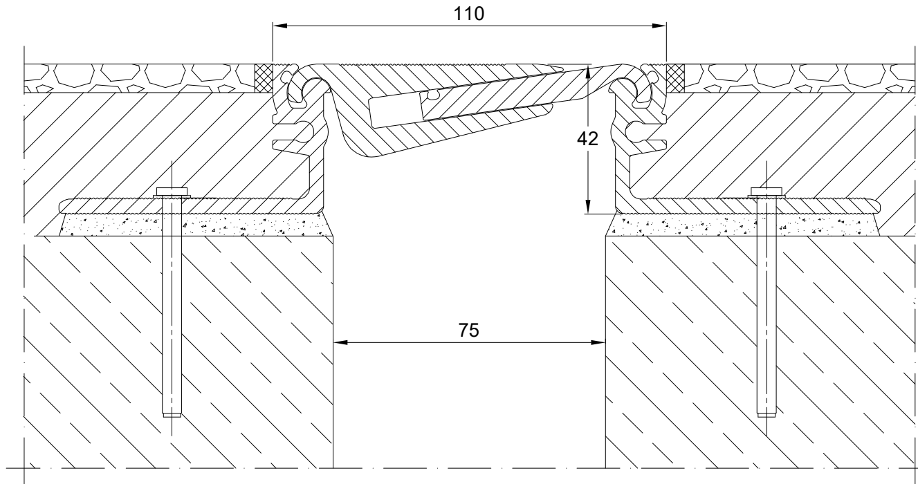
PROFIL DYLATACJNY AL 110.15.42 PRZEKRÓJ
