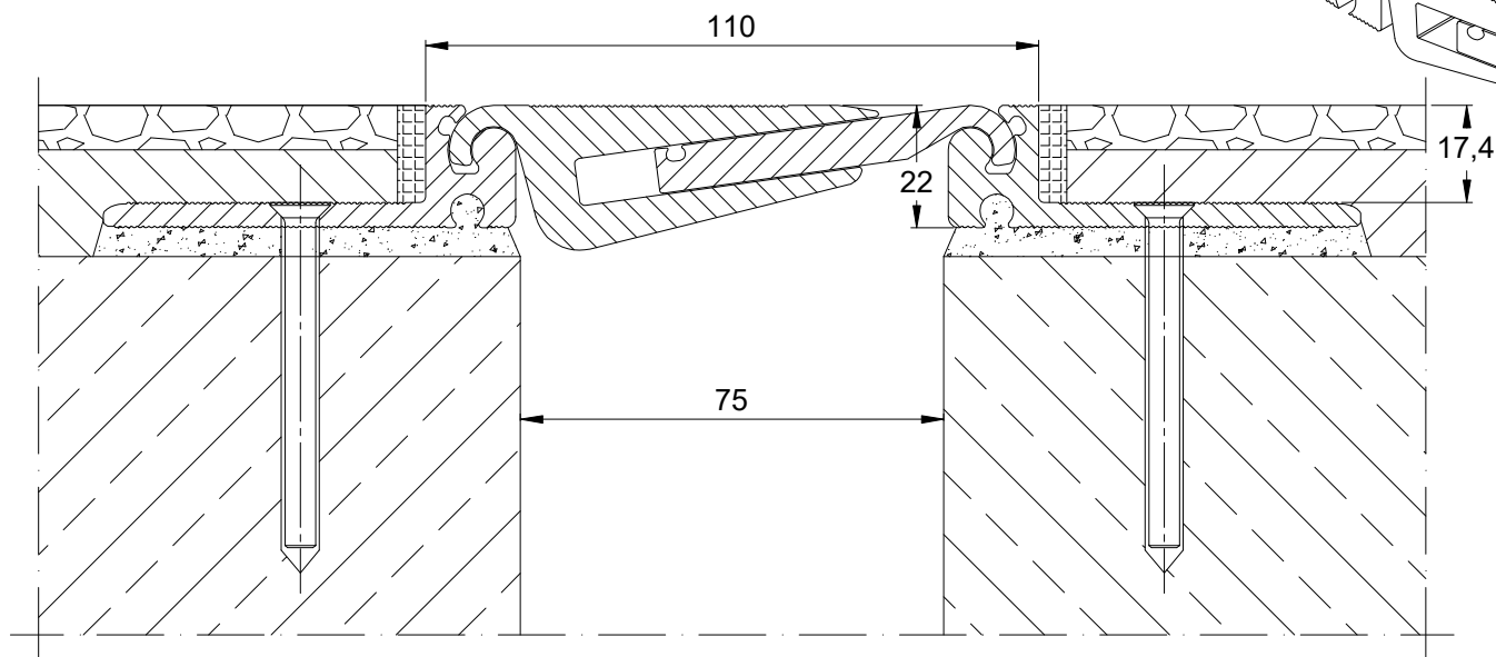
CONECTO AL 110.15.22 PRZEKRÓJ
