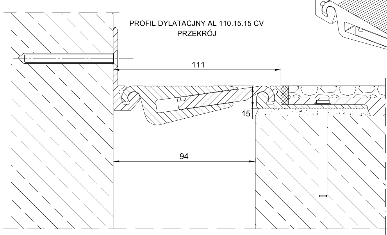
Profil dylatacyjny Conecto AL 110.15.15 CV
