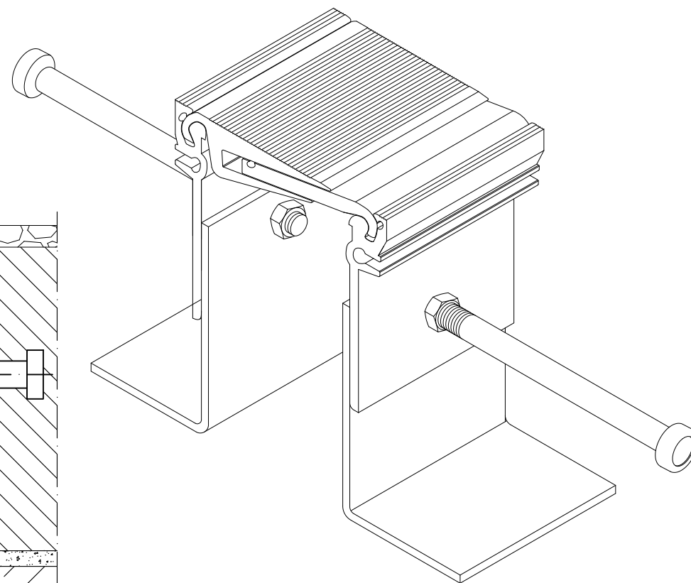
CONECTO AL 110.15.120& Rzut aksonometryczny
