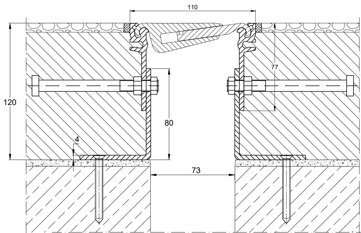
CONECTO AL 110.15.120& Przekrój
